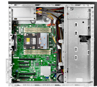
서버 내부
