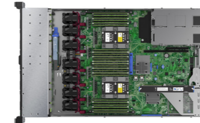
서버 내부
